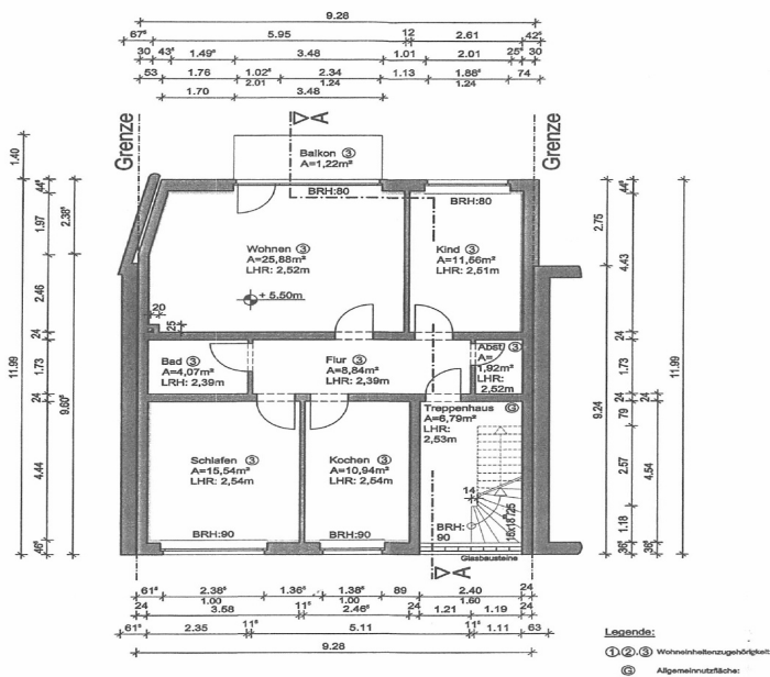
2. Obergeschoss
