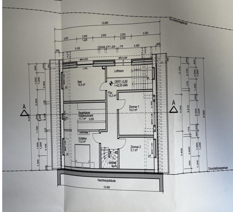
Grundriß Dachgeschoß
