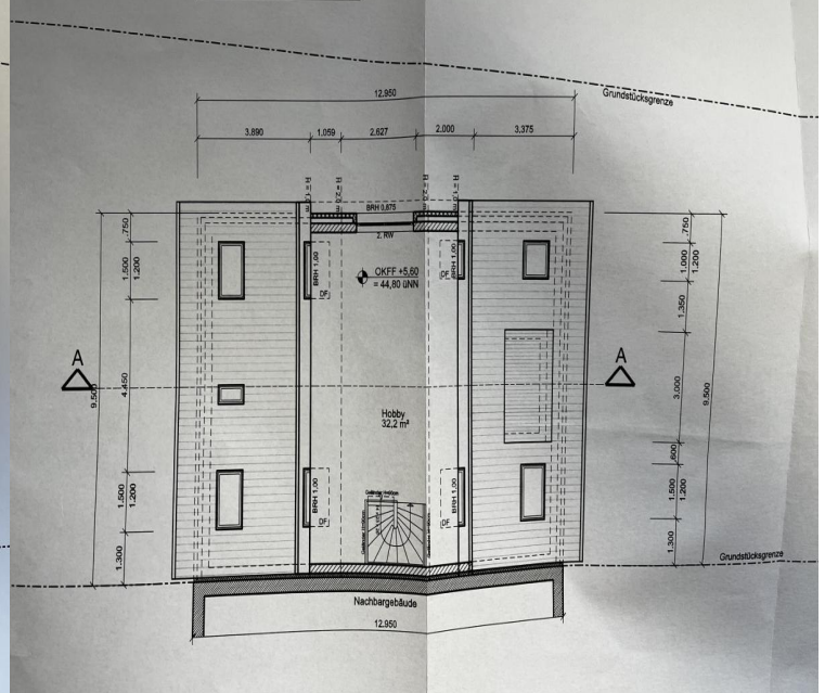
Grundriß Spitzboden
