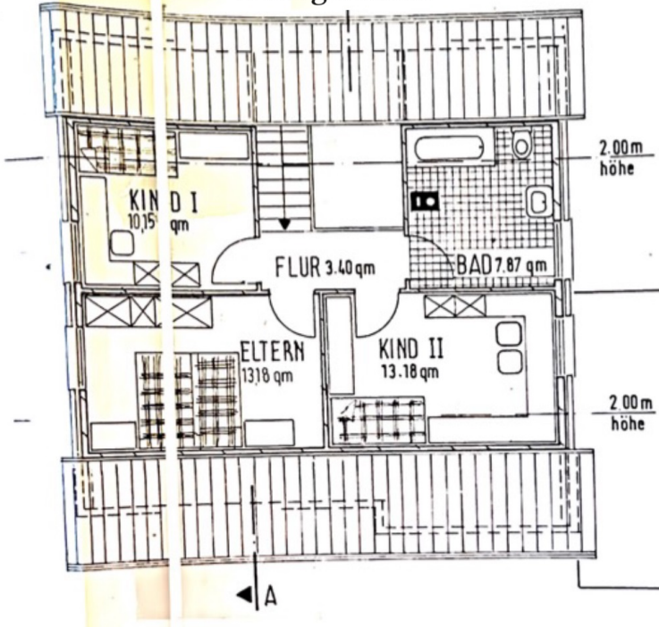
Dachgeschoss
